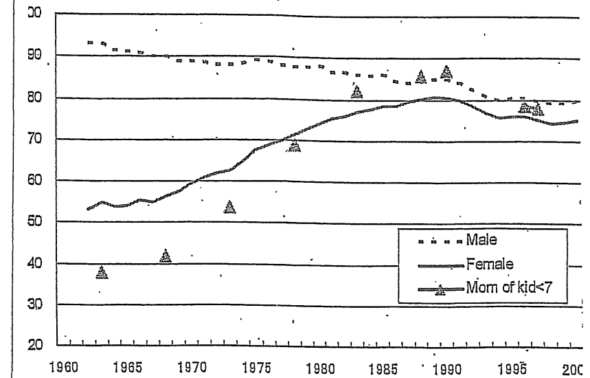
第二図 15~64歳の男女労働力率の推移：スウェーデン1960~2000
